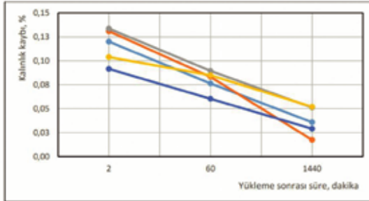
Şekil 3. Numunelerin kalınlık kaybı grafiği
